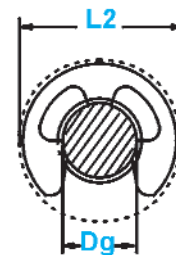
Diámetro límite instalado en la ranura
