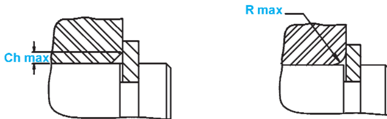
Radio y bisel de esquina máximos
