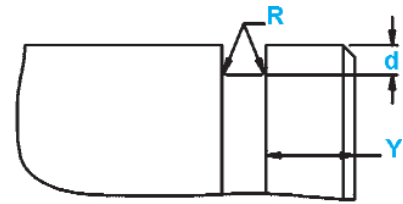
Vista desarrollada del perfil de ranura y margen del borde (Y) Radio interior máximo (R), esquinas pronunciadas para anillos 4 a 6; 0,005 para tamaños SE9 a 25; 0,010 para tamaños SE-31 a SE-43; 0,015 para tamaños 50 a SE-137
