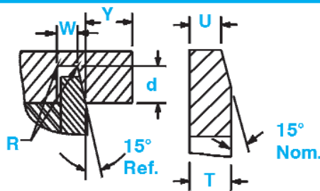
Vista desarrollada del perfil de ranura y margen del borde (Y) Radios inferiores máximos (R), 0,005 para tamaños de anillo -100 a -200; 0,010 para tamaños de anillo -206 a -1000
