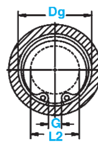
Diámetro límite y distancia de separación liberados en la ranura
