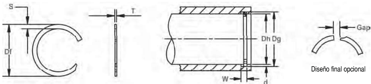
Diámetro de la carcasa y dimensiones de la ranura
