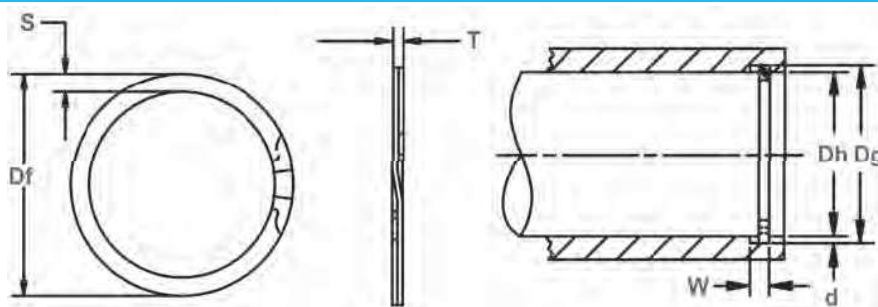
Diámetro libre y las mediciones del anillo
