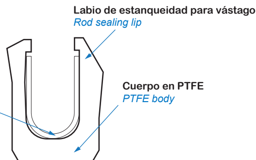
Muelle en acero inoxidable Stainless steel spring
